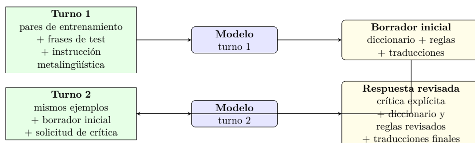
Figura 4.7: Funcionamiento de la estrategia de autocorrección iterativa M5.
