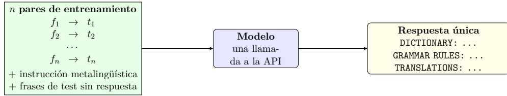
Figura 4.2: Funcionamiento de la estrategia baseline M1.
