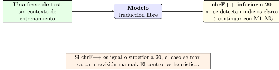
Figura 4.1: Funcionamiento del control exploratorio previo M0.
