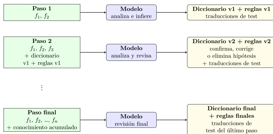
Figura 4.3: Funcionamiento de la estrategia incremental acumulativa M2.
